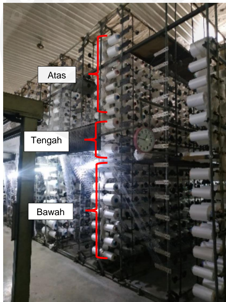
Lampiran 3. Creel pada mesin rajut lusi jacquard karl mayer RJSC 4 F NE dengan nomor mesin 91
