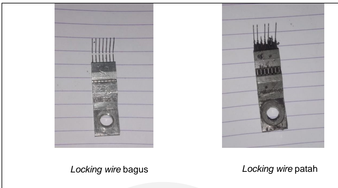
Lampiran 3 Perbedaan gambar Locking wire yang bagus dengan yang rusak
